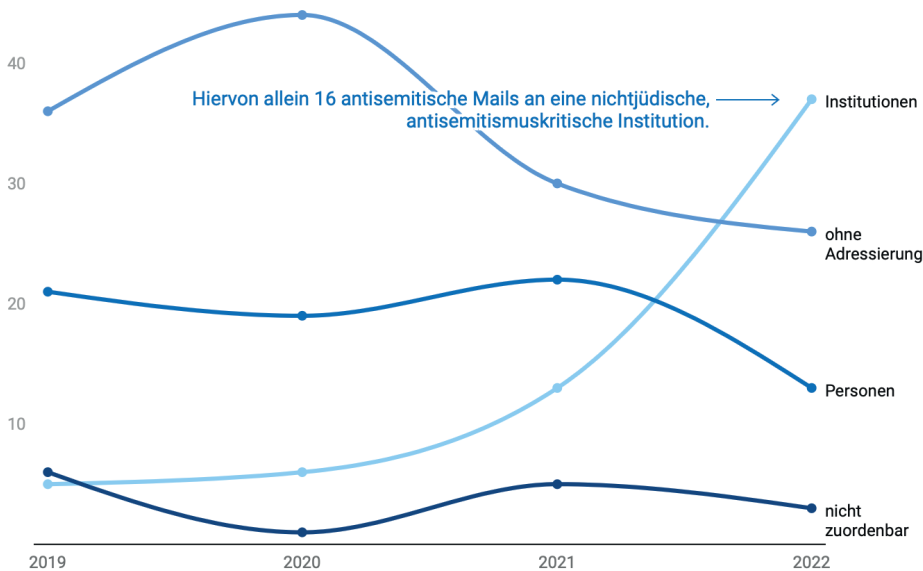
ADRESSIERUNG 2019–2022
