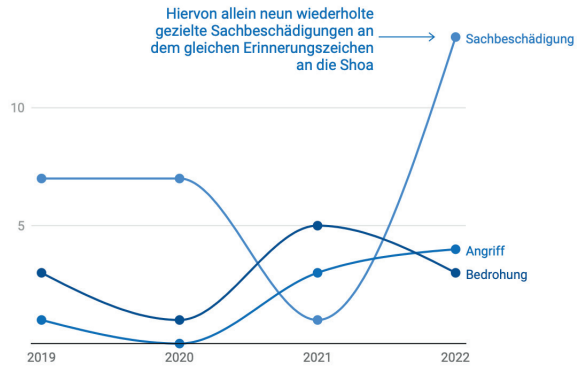
DELIKTQUALITÄT (AUSGEWÄHLT) 2019–2022
